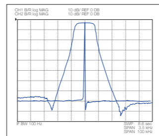
Esempio con caratteristica roofing-filter BW=500Hz
