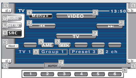
Schermo di controllo TV
